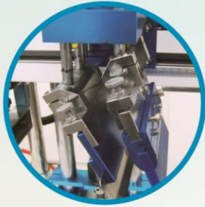
▲ 氣壓式刮膠座組直線升降
